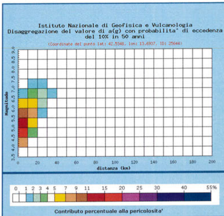
Fig. 2.7: Grafico di disaggregazione del valore di a(g) con probabilità di eccedenza del 10% in 50 anni, in termini di distanza epicentrale e magnitudo.
