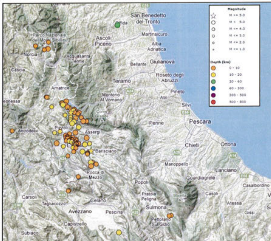
Fig. 2.2: Localizzazione eventi sismici dal 2007 ad oggi, con Magnitudo > 3.5, tratti dal catalogo di sismicità strumentale ISIDE ( http://iside.rm.ingv.it/iside/standard/index.jsp )
